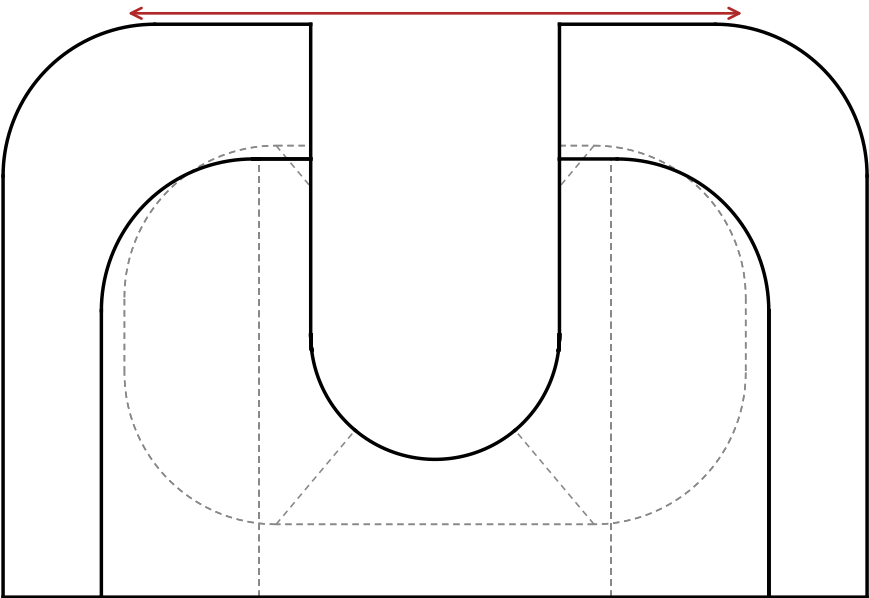
Вид с торца (Y-Z, сечение гнезда)
