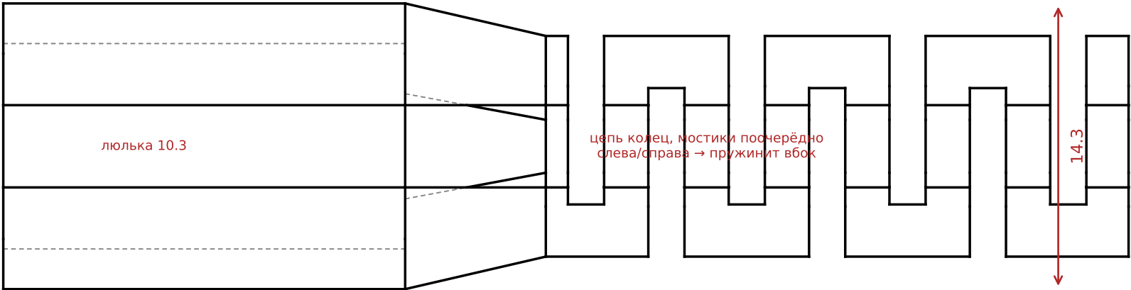
Вид сверху (X-Y): гнездо + серпантин (мостики L/R)
