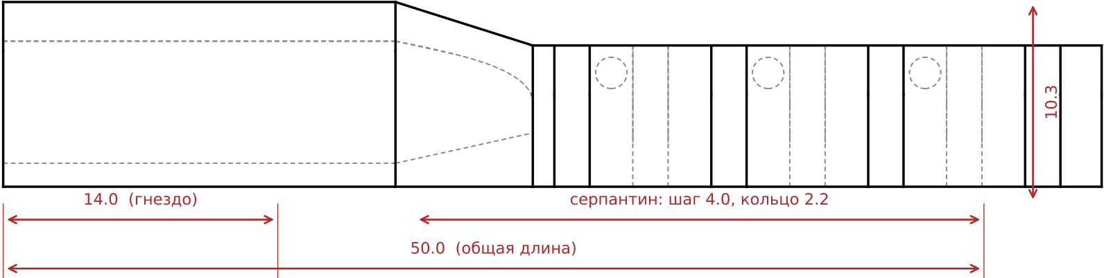
Вид сбоку (профиль X-Z)
